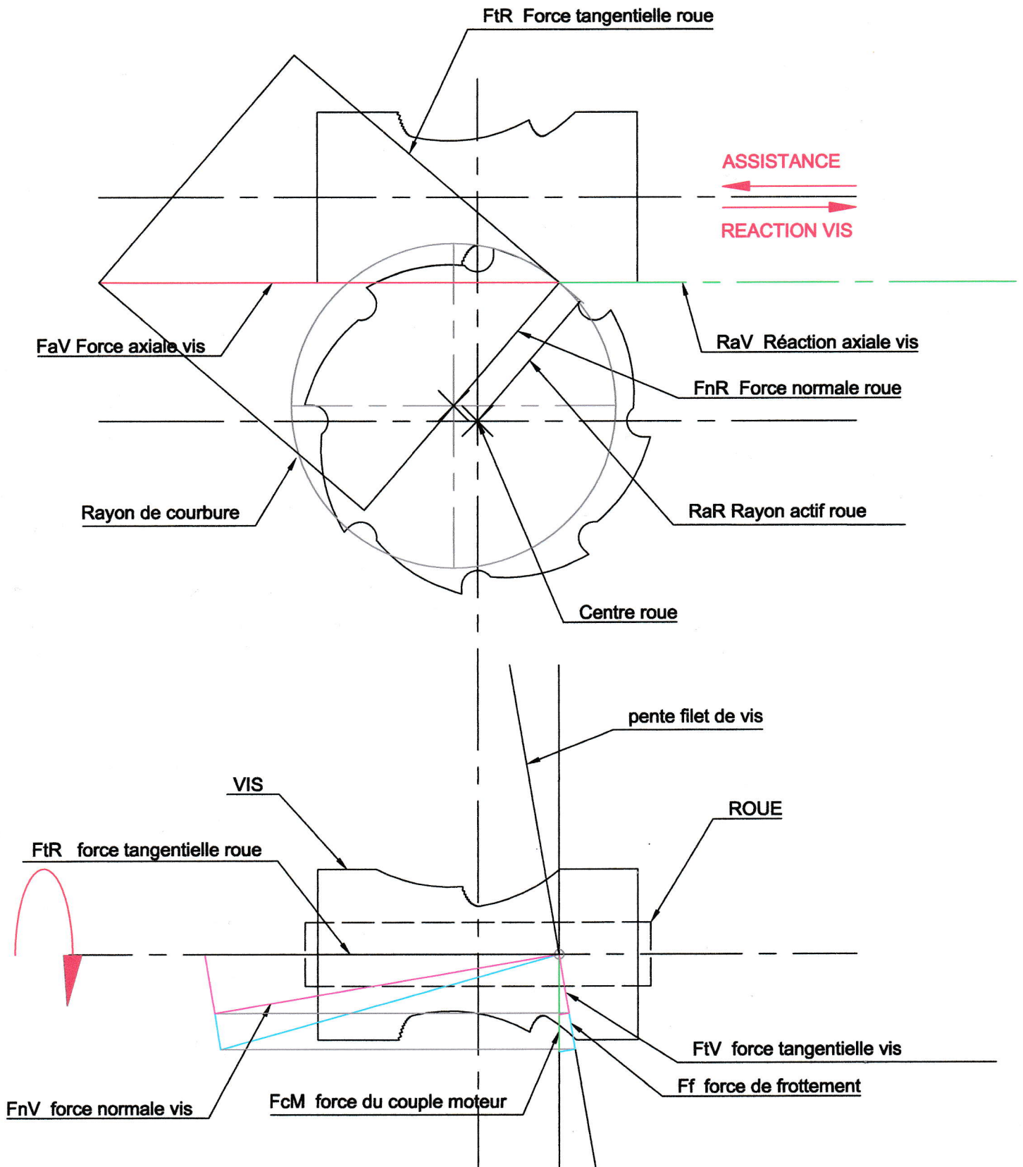
Représentation dans le plan commun roue-vis
